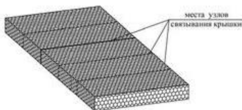
Рис. 6.11 Связывание крышки матрасно-тюфячных ГСИ
