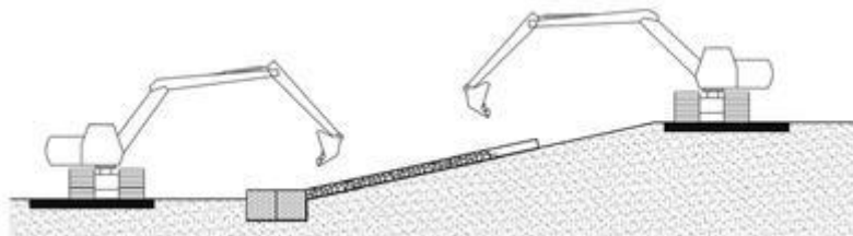
Рис. 6.5 Заполнение матрасно-тюфячных габионов механизированным способом
