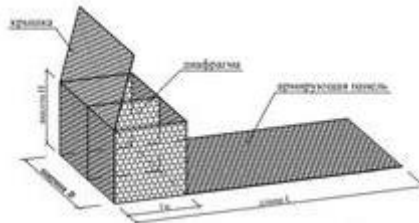
Рис. 7.1 Конструктивная схема коробчатых габионов с армопанелью
