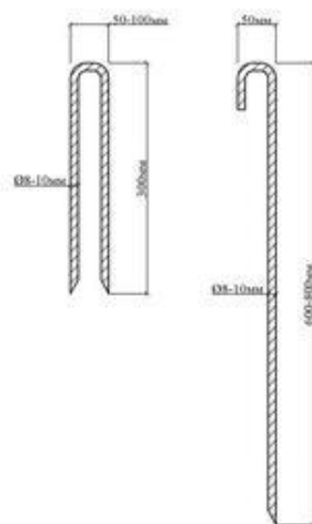
Рис. 6.8 Схема анкеровки матрасно-тюфячных ГСИ
