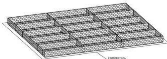
Рис. 6.4 Несколько связанных вместе матрасно-тюфячных габионов
