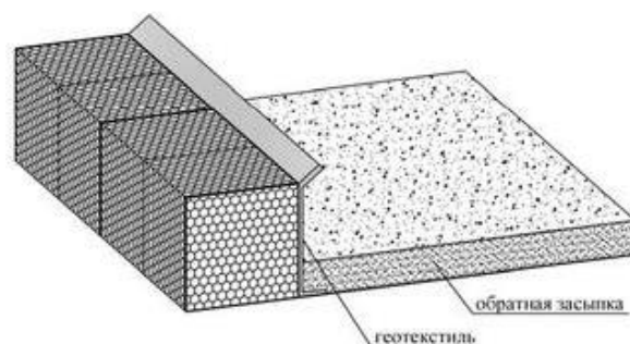
Рис. 7.8 Послойная обратная засыпка армирующей панели
