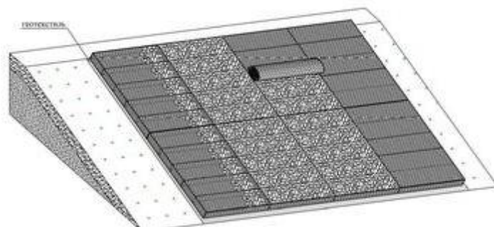
Рис. 6.10 Установка крышки матрасно-тюфячных габионов на всю длину укрепления
