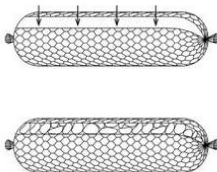
Рис. 8.4 Заполнение камнем цилиндрической габионной конструкции
