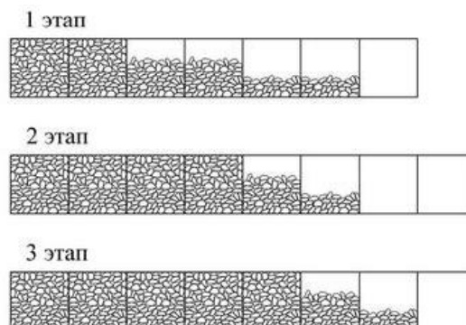
Рис. 5.12 Последовательность заполнения коробчатых габионных конструкций
