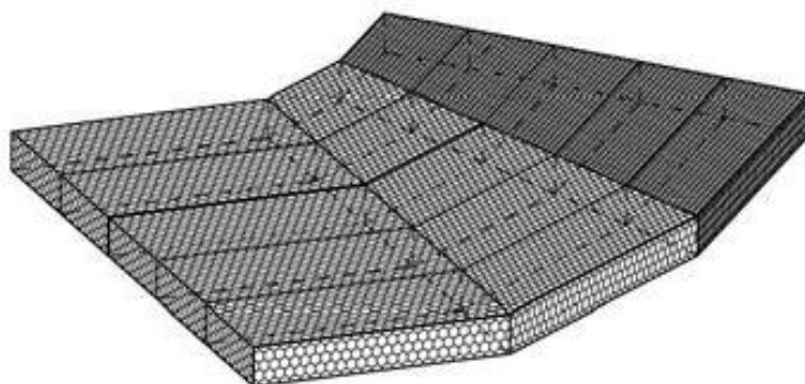
Рис. 6.12 Резка матрасно-тюфячных габионных конструкций
