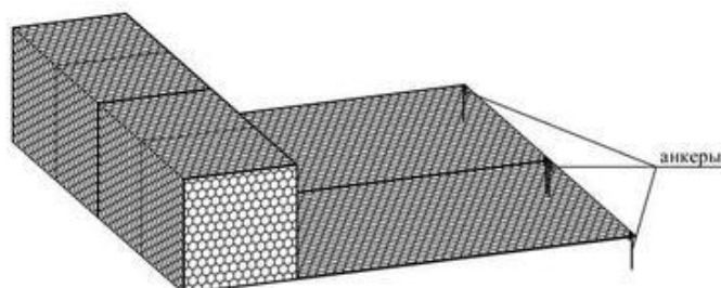
Рис. 7.7 Установка анкеров по краям армирующей панели
