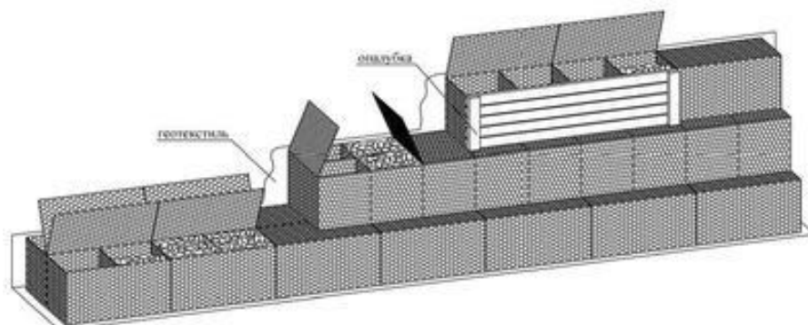
Рис. 5.8 Формирование сооружения из коробчатых габионных изделий
