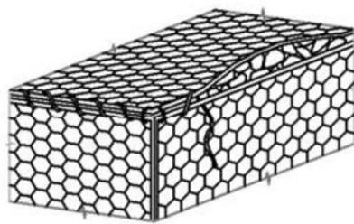
Рис. 5.15 Установка крышки габиона
