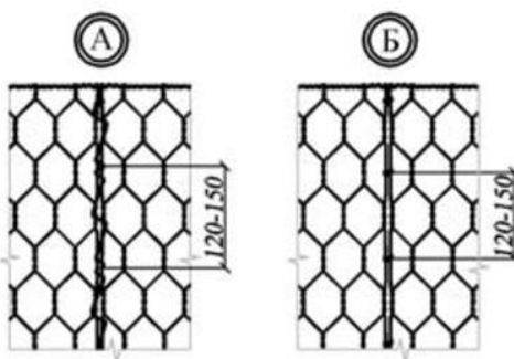
Рис. 5.6 Перевязка элементов габиона
