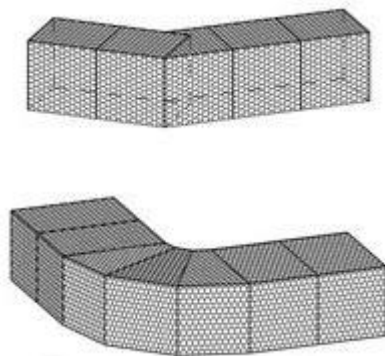
Рис. 5.16 Резка коробчатых габионов при создании пологого закругления сооружения
