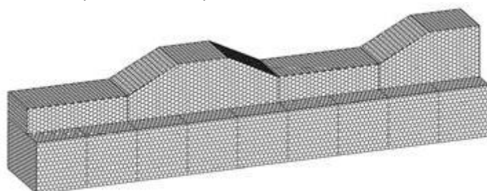
Рис. 5.18 Подпорная стена из коробчатых габионов с плавной траекторией
