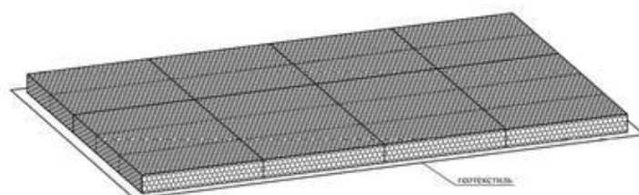
Рис. 6.9 Установка крышки матрасно-тюфячных габионных конструкций
