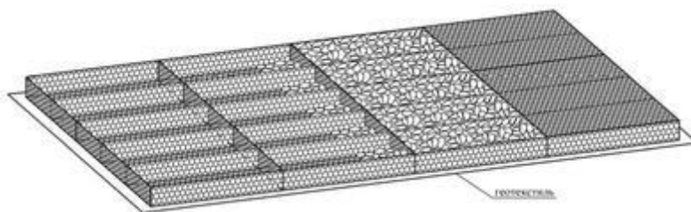
Рис. 6.6 Формирование сооружения из матрасно-тюфячных ГСИ
