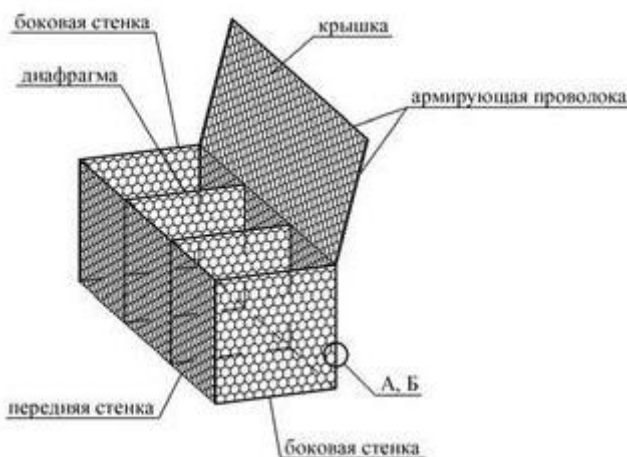
Рис. 5.5 Собранный коробчатая габионная конструкция
