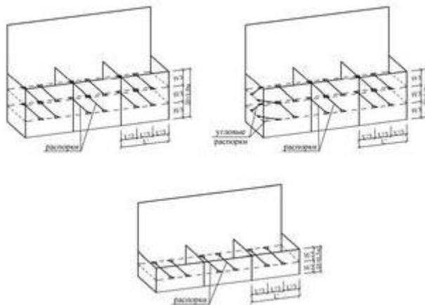
Рис. 5.13 Схема устройства распорок в коробчатых габионах высотой 0,5 и 1,0 м
