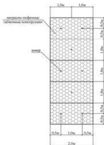
Рис. 6.8 Схема анкеровки матрасно-тюфячных ГСИ
