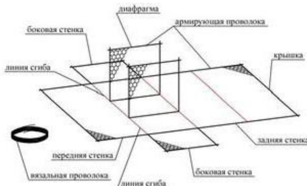
Рис. 5.4 Установка диафрагм в коробчатой габионной конструкции
