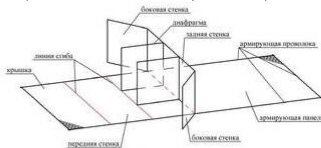
Рис. 7.2 Развертка коробчатого габиона с армирующей панелью
