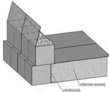
Рис. 7.9 Установка вышележащих коробчатых габионных конструкций с армирующей панелью
