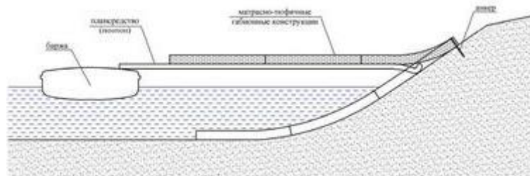
Рис. 6.14 Погрузка матрасно-тюфячных габионов, заполненных камнем, под воду при помощи плавсредств
