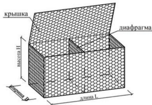
Рис. 5.1 Элементы коробчатого габиона
