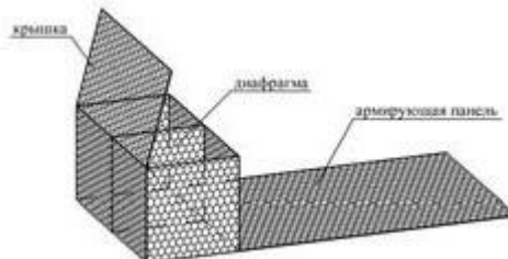
Рис. 7.3 Собранная коробчатая габионная конструкция с армирующей панелью
