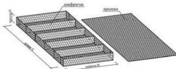
Рис. 6.1 Конструктивная схема габионных конструкций матрасно-тюфячного типа
