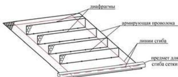
Рис. 6.2 Развертка матрасно-тюфячного габиона
