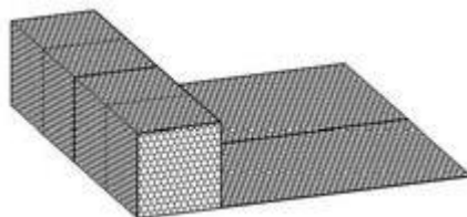
Рис. 7.6 Установка крышки коробчатых габионных конструкций с армопанелью
